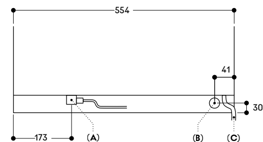
A: Morsetteria elettrica B: Scarico acqua C: Carico acqua fredda
