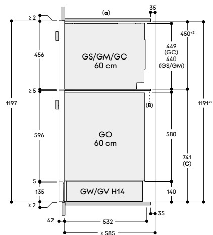
Vista laterale
