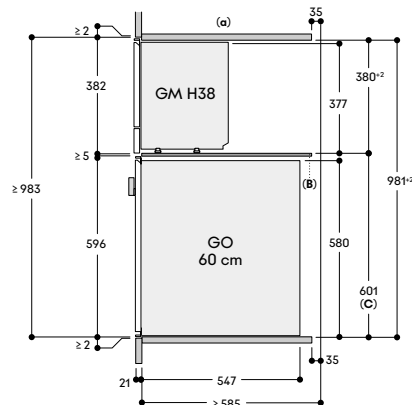
Vista laterale
