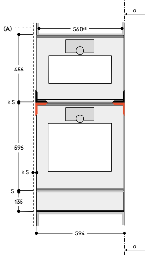
Vista frontale
